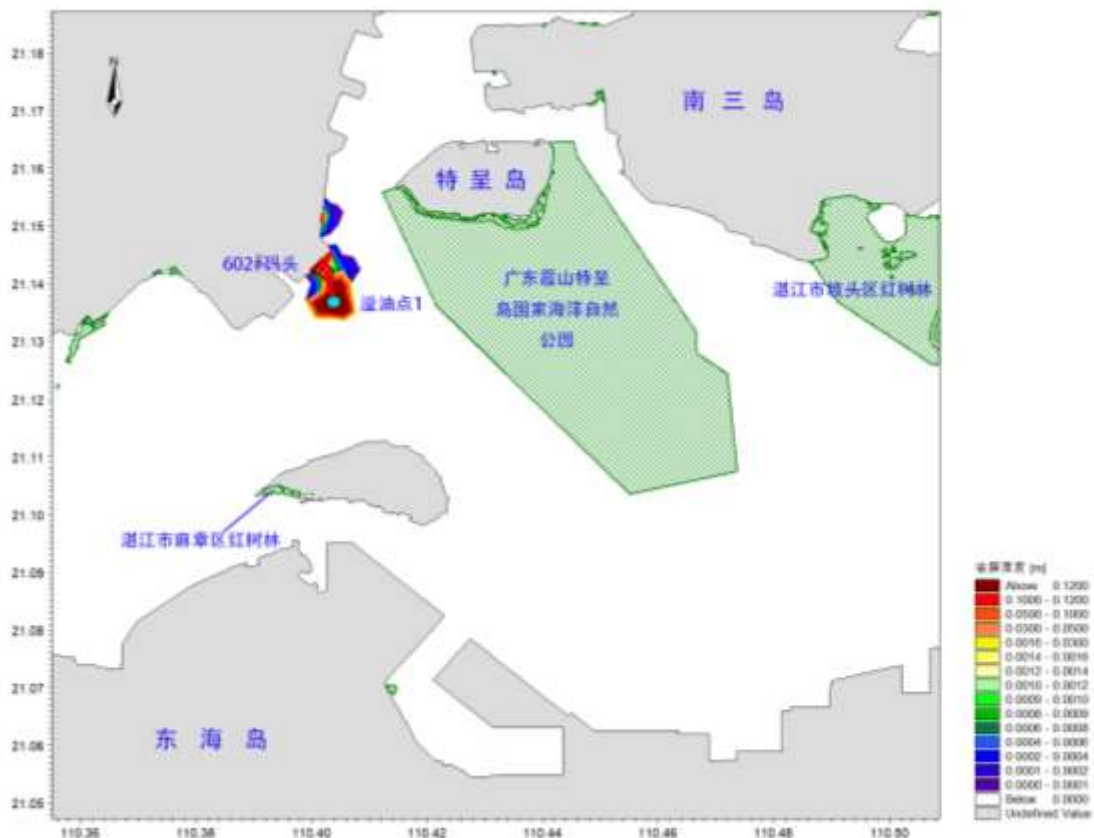
图 8.5-14 72h 扫海范围（码头前沿/涨潮 SE）
