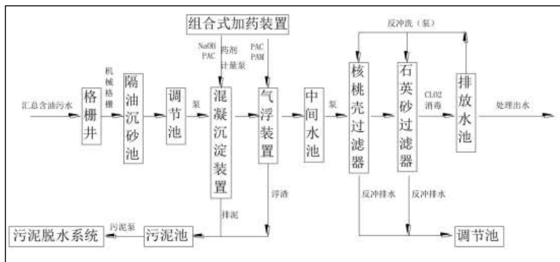
图 9.2-1 含油废水预处理工艺流程图
