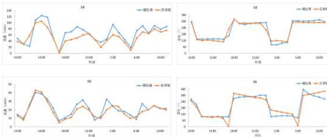
图 8.5-5 S1、S3、S4、S6 流速、流向验证
