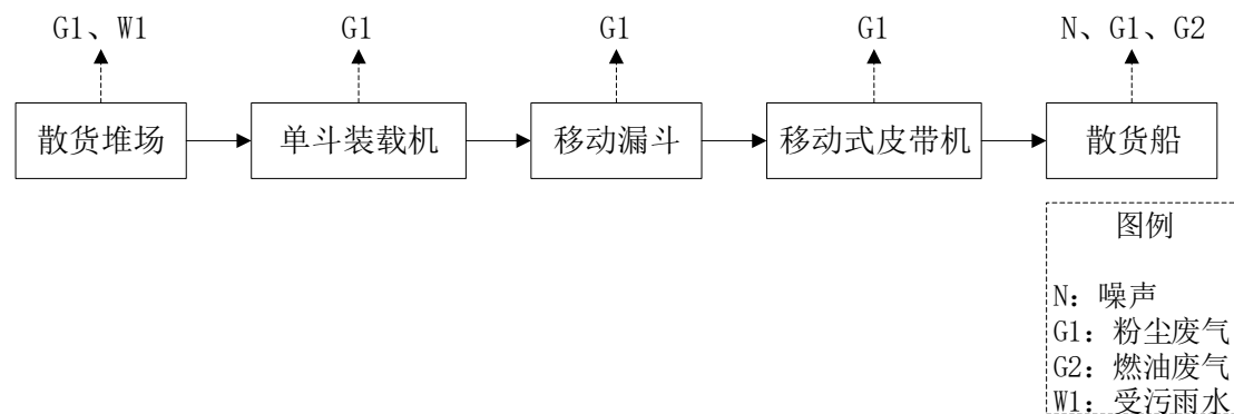
图 3.5-1 现有项目装卸工艺流程以及产污环节图
