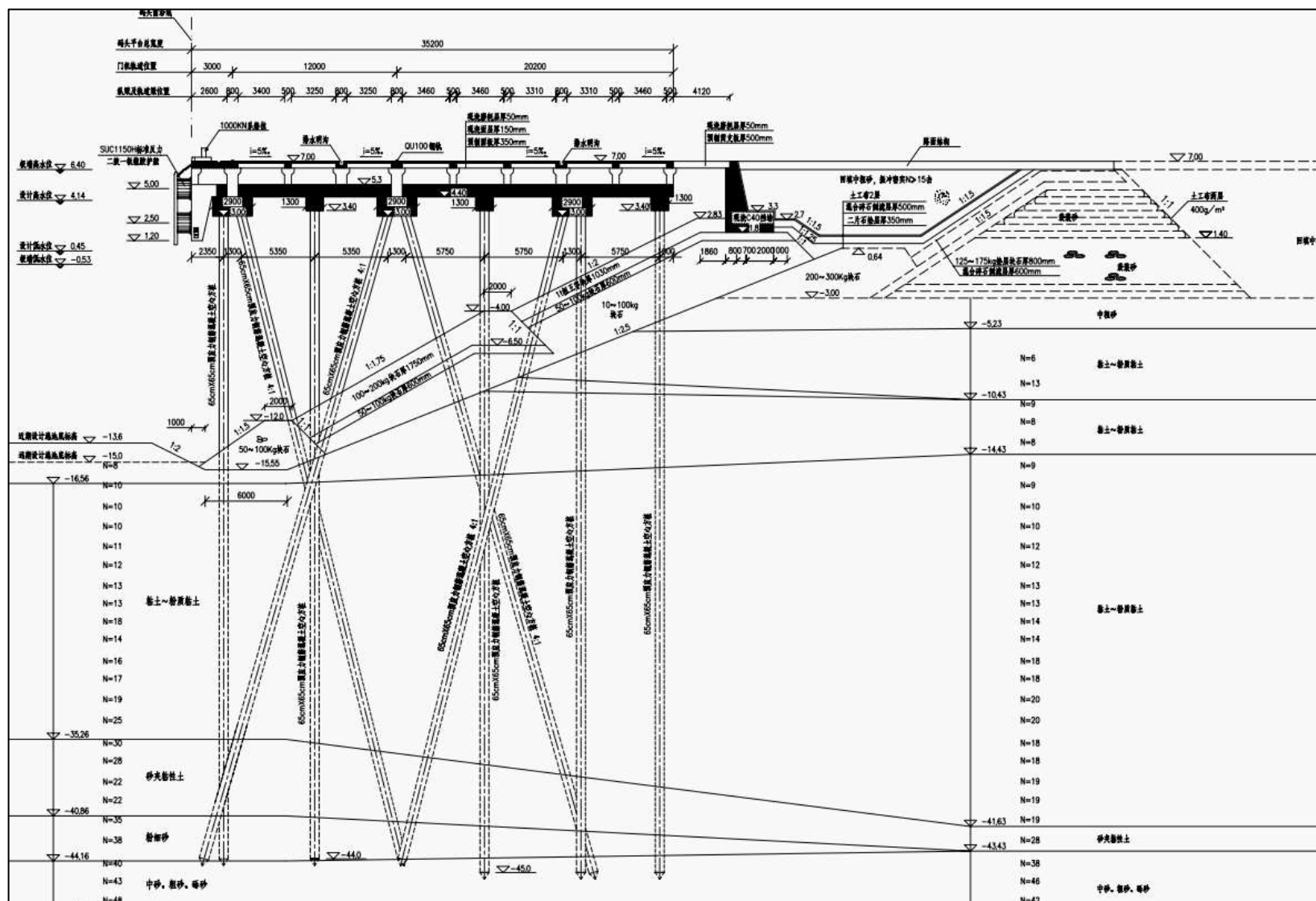
图 3.2-4 602#泊位结构断面图
