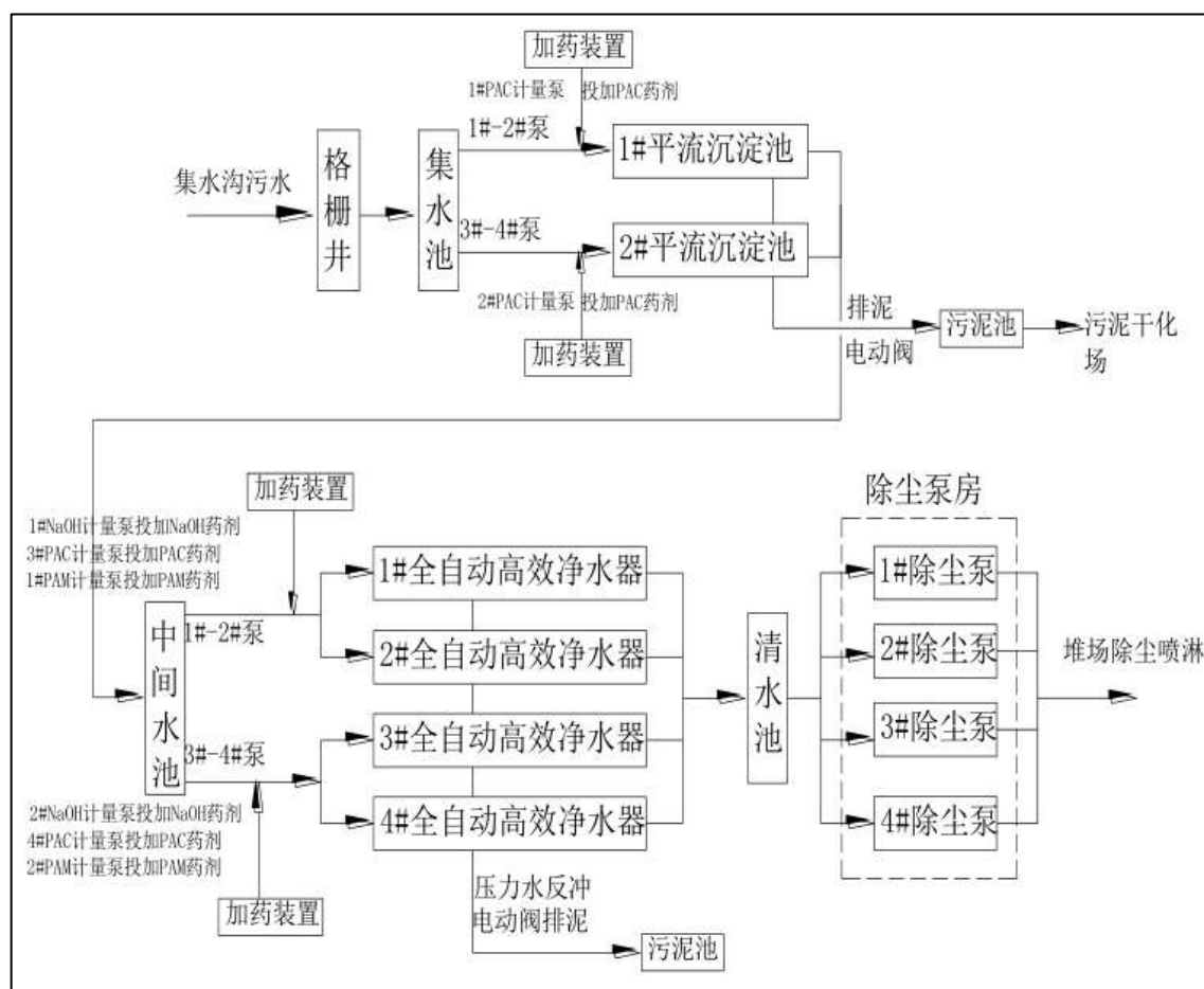
图 9.2-3 含矿废水处理工艺流程图
