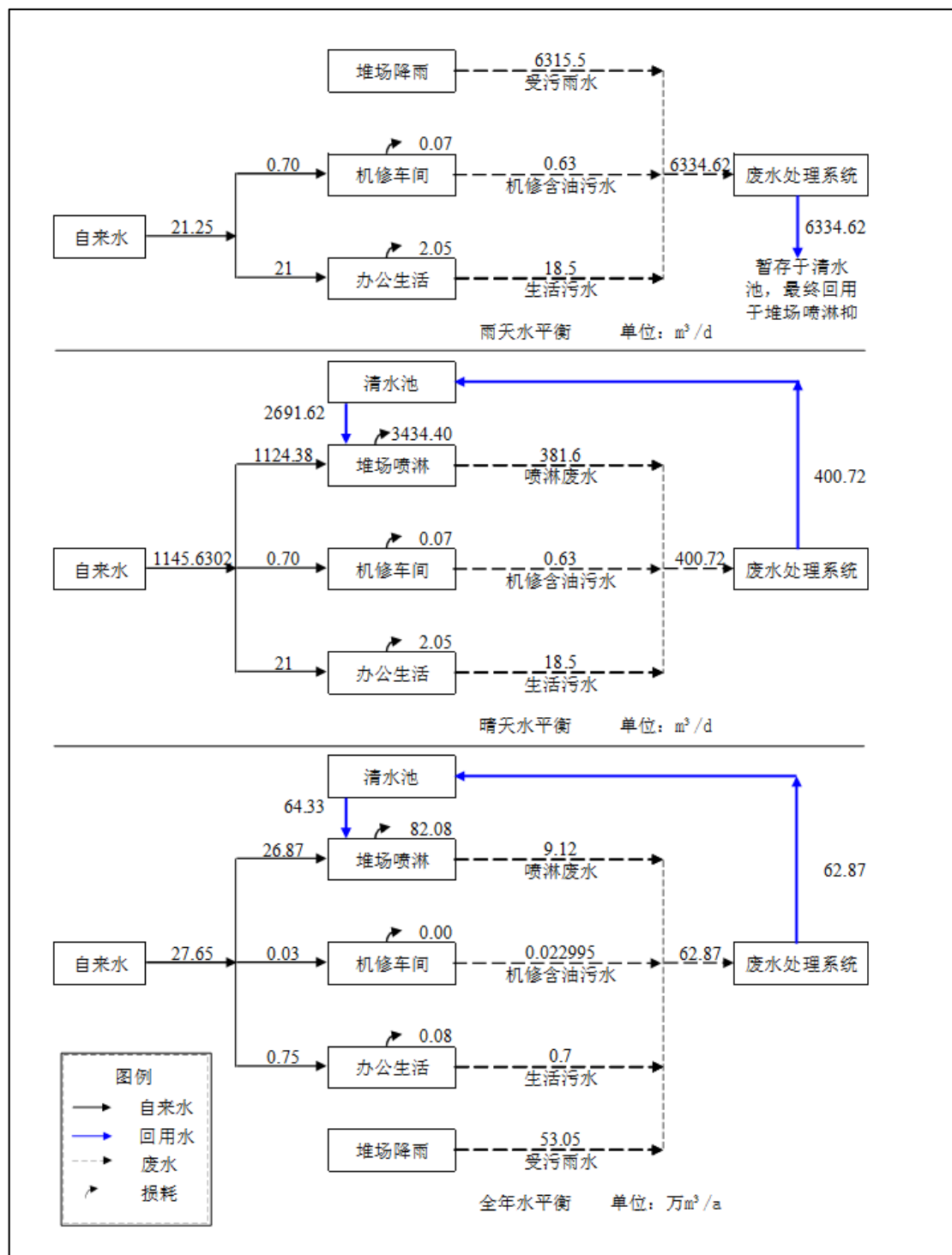
图 4.3-1 本项目水平衡图
