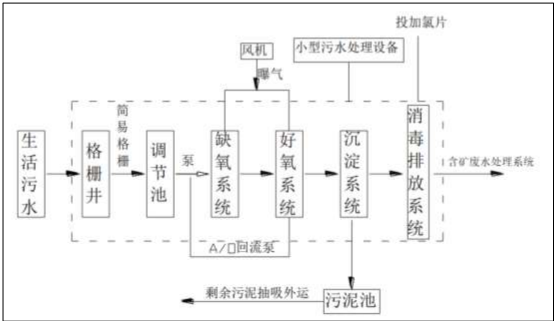
图 3.5-2 生活污水预处理工艺流程图
