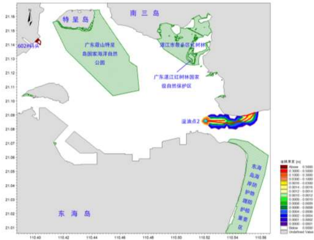
图 8.5-20 72h 扫海范围（航道相交处 1/落潮/SE）
