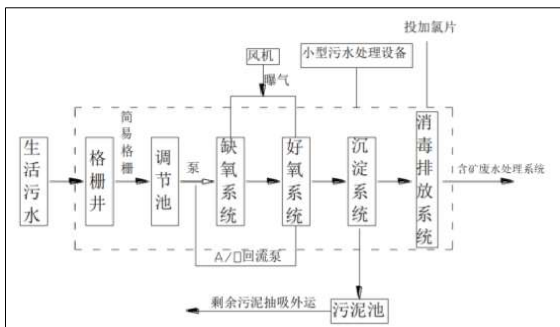
图 9.2-2 生活污水预处理工艺流程图
