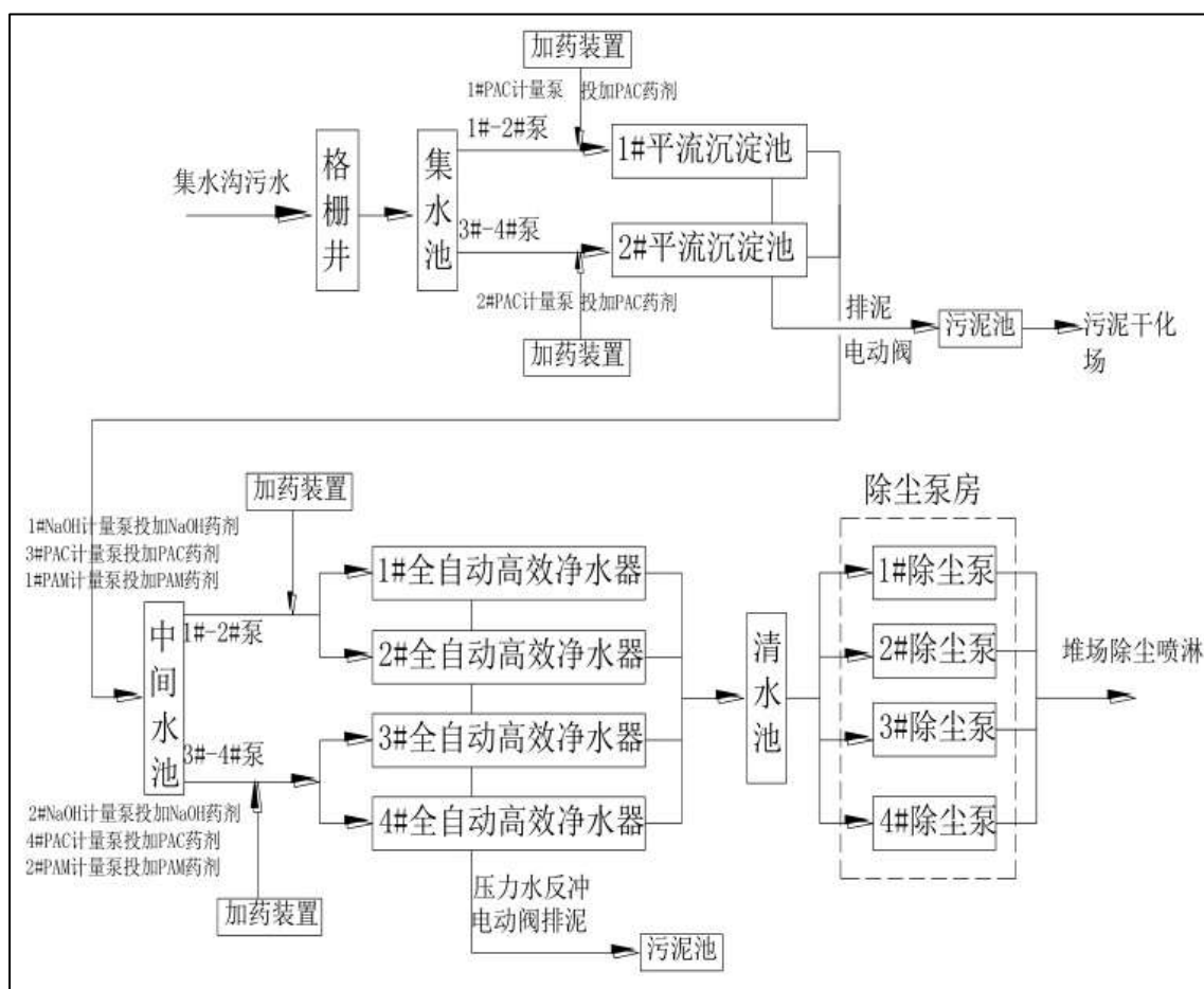
图 3.5-3 含矿废水处理工艺流程图
