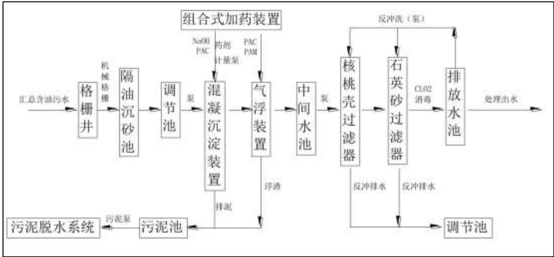
图 3.5-1 含油废水预处理工艺流程图
